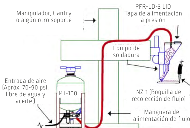
PT-100
